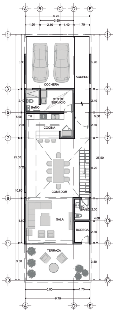
PLANTA ARQUITECTÓNICA BAJA
