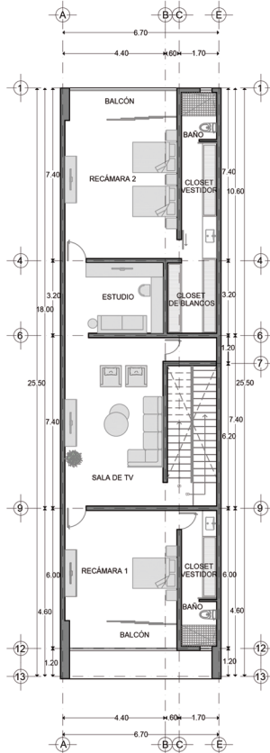
PLANTA ARQUITECTÓNICA ALTA
