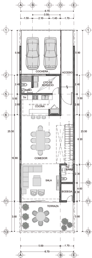
PLANTA ARQUITECTÓNICA BAJA
