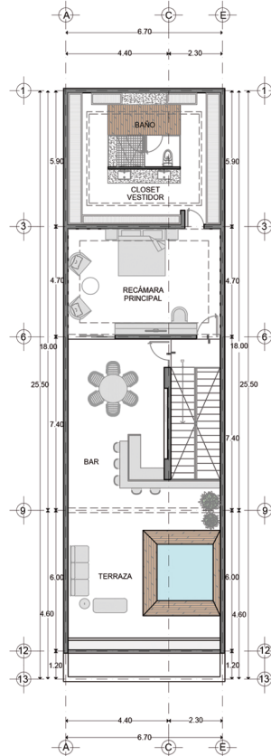
PLANTA ARQUITECTÓNICA TERCER NIVEL
